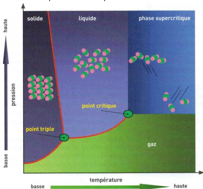
Diagramme de phases pression –température d'un corps pur.
